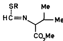
(14) R = Me
